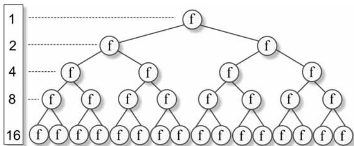
Рис. 18.5. Рекурсивное нахождение числа Фибоначчи
