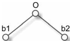
Рис. 18.2. Бинарное дерево
