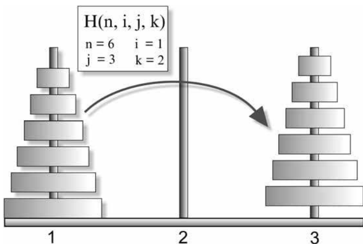
Рис. 18.3. Задача о ханойских башнях
